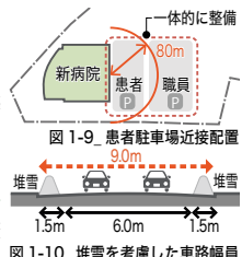
図 1-10 堆雪を考慮した車路幅員
